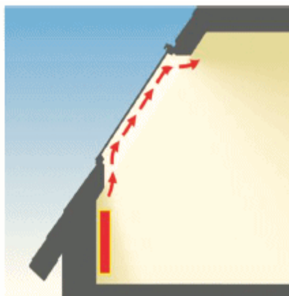
Рисунок 3 - Пример расположения мансардного окна относительно отопительных приборов
